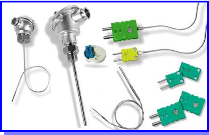
Sondes PT100, thermocouples, transmetteurs infra rouge.
